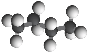
n - Butane - C 4 H 10
