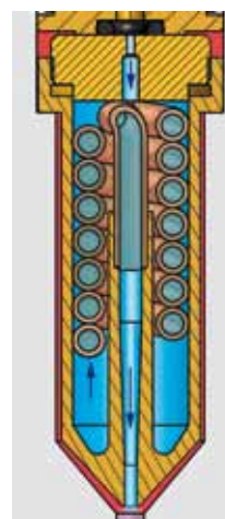
Abb.: Injektor
